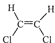
cis -1,2-đicloeten
