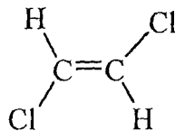
trans -1,2-đicloeten
